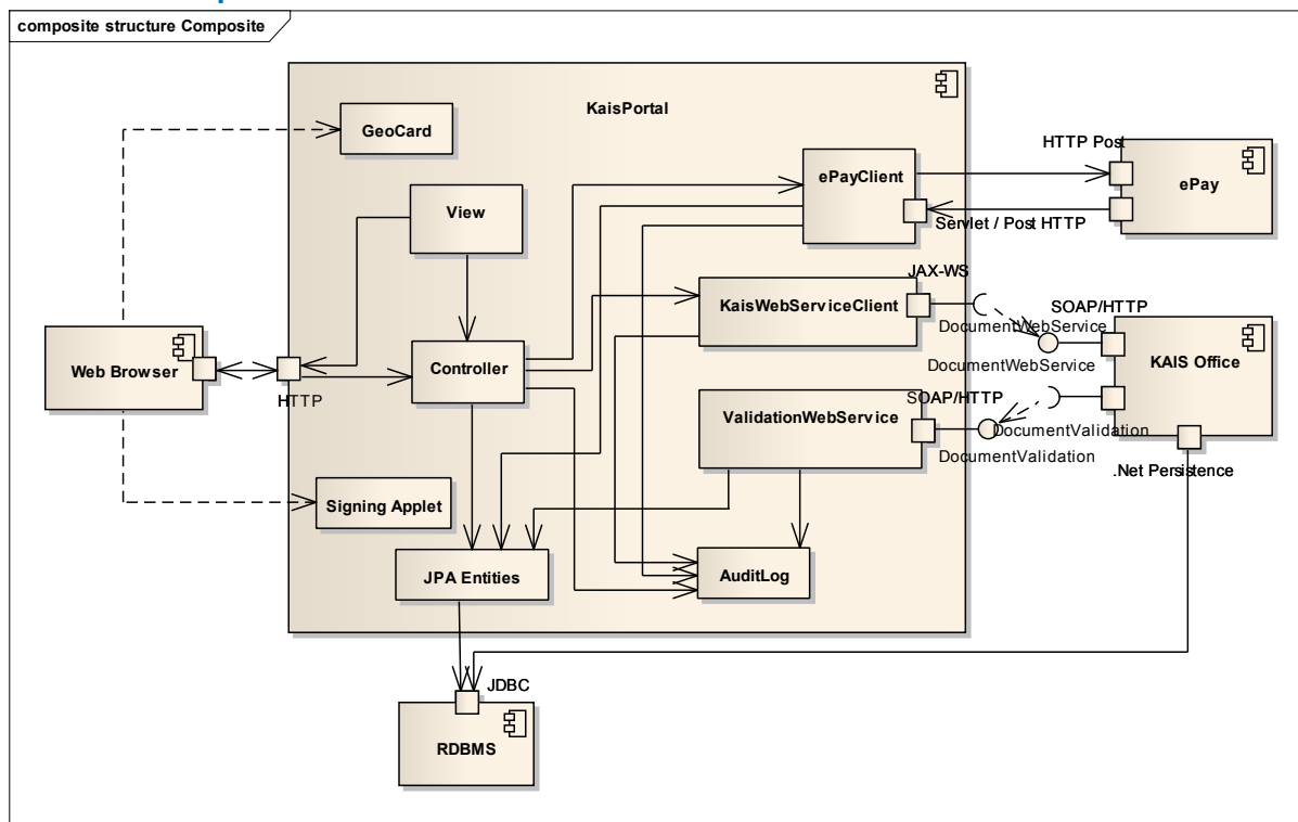
Фигура: Структура на КАИС Портал
