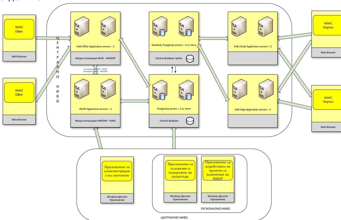
Фигура: Схема на архитектурата на ИИСКИР
